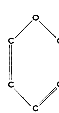
PYRAN
