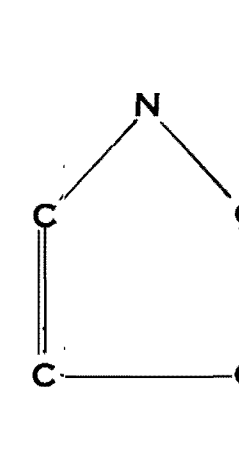
PYRROLE
